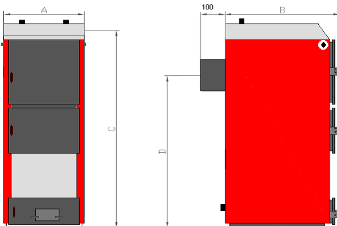
Rys. 2 Schemat poglądowy MINI
