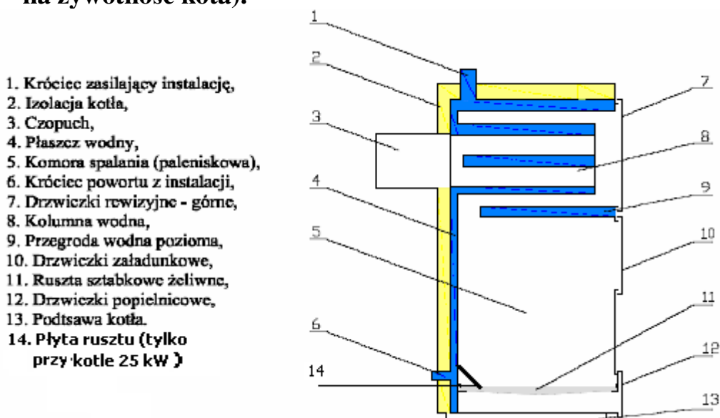
Rys. 1 Przekrój wzdłużny kotła MINI
