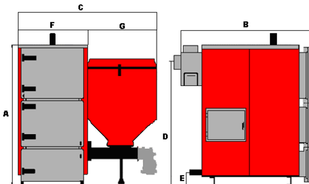
Rys. 2 Widok poglądowy kotła HEITZ MAX EKO
