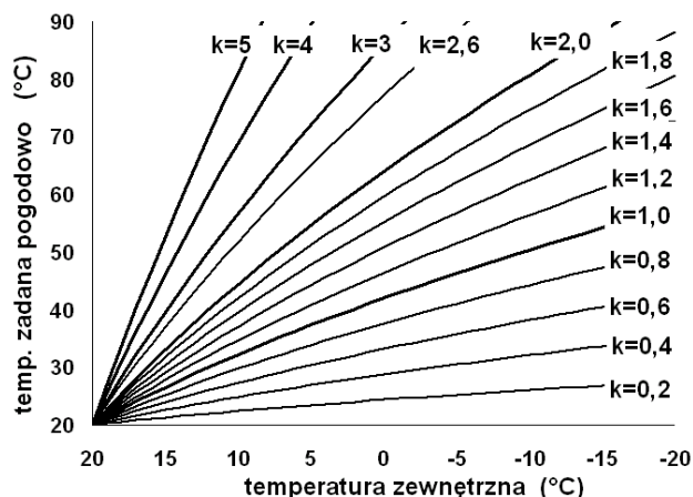
Rys. 15 Krzywe grzewcze
