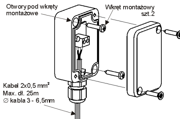
Rys. 32. Podłączenie czujnika pogodowego CT4-P, czujnik nie stanowi standardowego wyposażenia regulatora.
