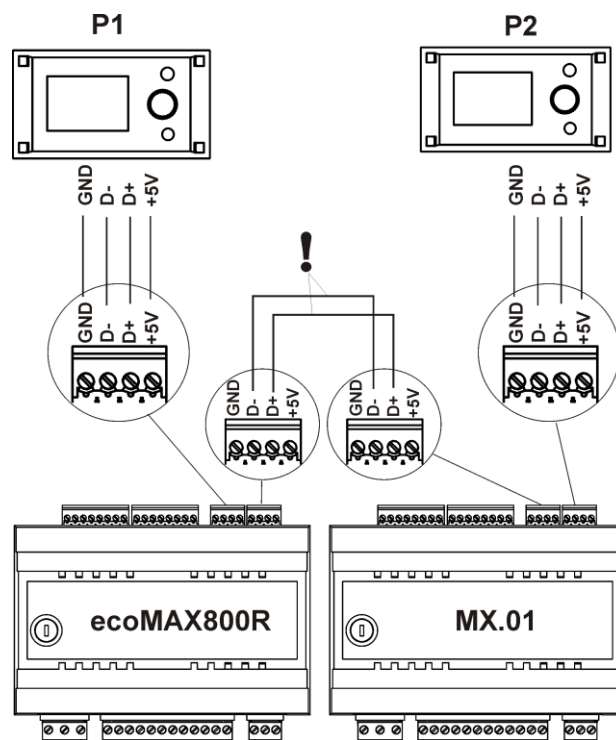
Rys. 42 Podłączenie panelu dodatkowego, gdy jest podłączony moduł rozszerzający mieszaczy MX.01,
