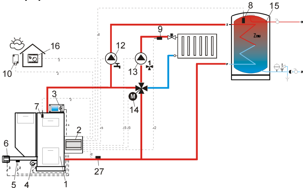
Rys. 21 Schemat z zaworem czterodrogowym sterującym obiegiem centralnego ogrzewania 2 , gdzie: 1 – kocioł z podajnikiem retortowym, 2 – regulator ecoMAX – moduł wykonawczy, 3 – regulator ecoMAX – panel sterujący, 4 – Wentylator, 5 – czujnik temperatury podajnika, 6- silnik motoreduktora, 7 – czujnik temperatury kotła, 8 – czujnik temperatury ciepłej wody użytkowej, 9 czujnik temperatury mieszacza, 10 – czujnik temperatury – pogodowy, 12 – pompa obiegu ciepłej wody użytkowej, 13 – pompa obiegu mieszacza, 14 – siłownik mieszacza, 15 – zasobnik ciepłej wody użytkowej, 16 – termostat pokojowy, 27 – czujnik temperatury powrotu.
