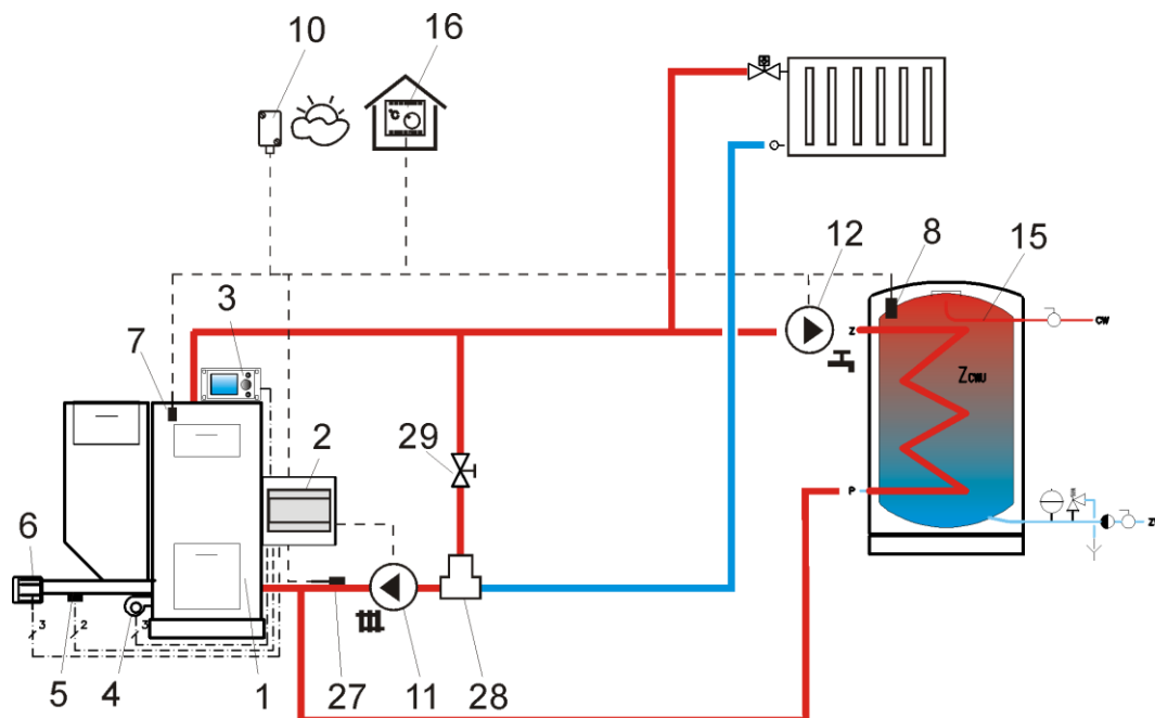
Rys. 22 Schemat z termostatycznym zaworem trójdrogowym chroniącym temperaturę wody powrotnej 3 , gdzie: 1 – kocioł z podajnikiem retortowym, 2 – regulator ecoMAX – moduł wykonawczy, 3 – regulator ecoMAX – panel sterujący, 4 – wentylator, 5 – czujnik temperatury podajnika, 6- silnik motoreduktora, 7 – czujnik temperatury kotła, 8 – czujnik temperatury ciepłej wody użytkowej, 9 czujnik temperatury mieszacza, 10 – czujnik temperatury – pogodowy, 11 – pompa obiegu centralnego ogrzewania, 12 – pompa obiegu ciepłej wody użytkowej, 13 – pompa obiegu mieszacza, 15 – zasobnik ciepłej wody użytkowej, 16 – termostat pokojowy, 27 – czujnik temperatury powrotu, 28 – termostacyjny zwór trójdrogowy 50-55°C, 29 – zawór dławiący (grzybkowy).
