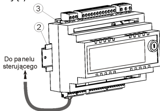
Rys. 27 Osadzenie regulatora na szynie, gdzie: 1- moduł wykonawczy, 2 - szyna DIN TS35, 3 - zaczepty.
