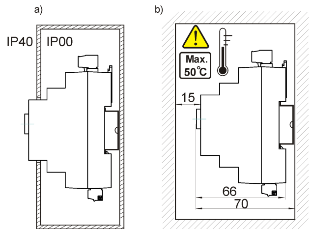
Rys. 29 Metody zabudowy modułu: a - w obudowie modułowej z dostępem do powierzchni czołowej, b - w obudowie bez dostępu do powierzchni czołowej.
