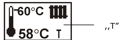
Rys. 34 Widok okna głównego po zadziałaniu termostatu
