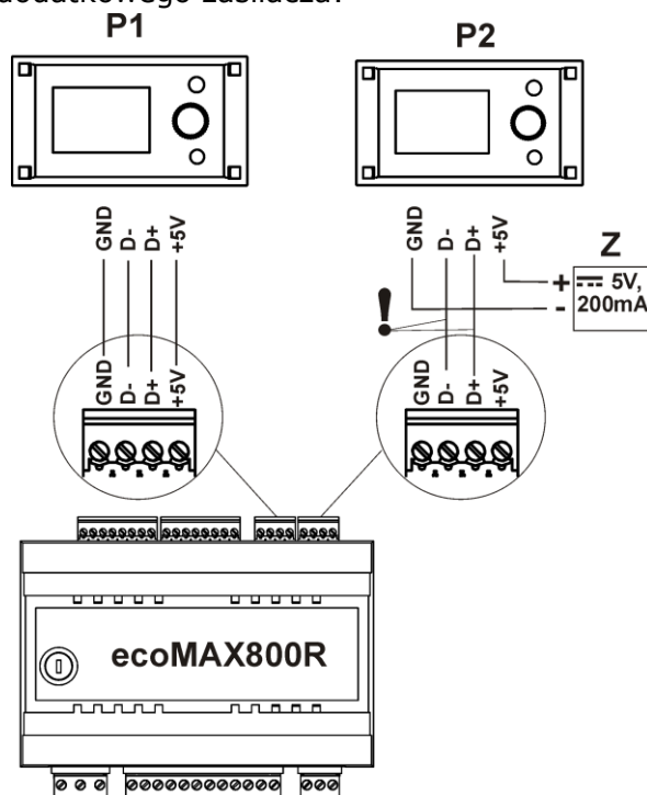
Rys. 41 Podłączenie panelu dodatkowego, gdy nie jest podłączony moduł mieszaczy MX.01, gdzie: P1 – panel kotła, P2 – panel w pomieszczeniach mieszkalnych, Z – zasilacz, ! – łączyć dwuprzewodowo.
