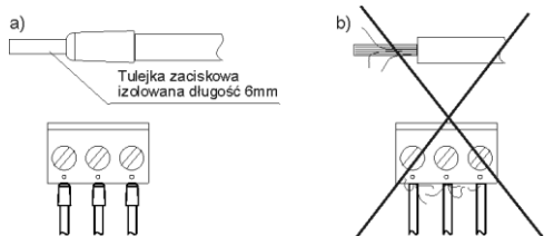
Rys. 30 Zabezpieczanie końców przewodów: a) prawidłowe, b) nieprawidłowe
