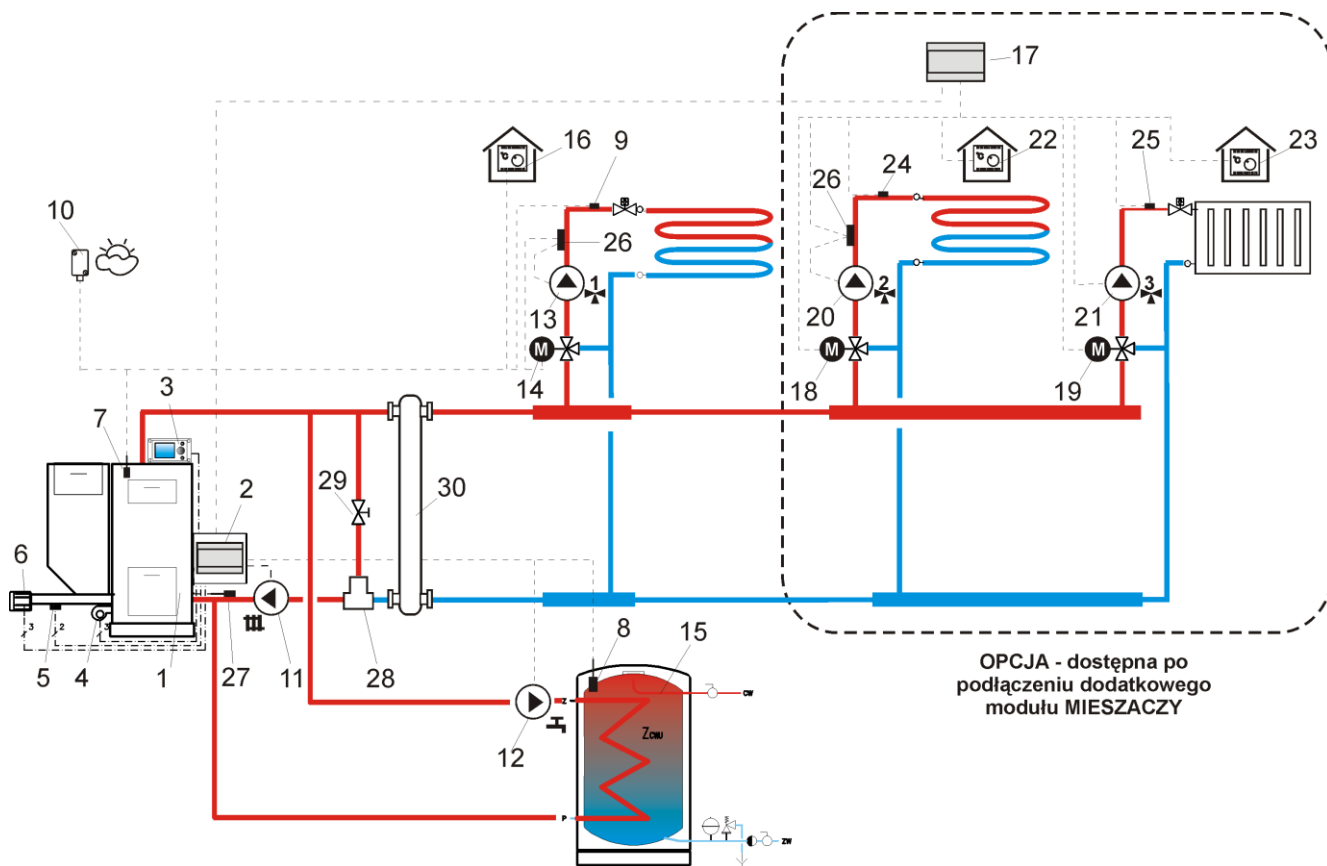
Rys. 23 Schemat z termostatycznym zaworem trójdrogowym chroniącym temperaturę wody powrotnej i zaworem trójdrogowym zasilającym ogrzewanie podłogowe oraz z dwoma dodatkowymi obiegami mieszacza po podłączeniu modułu rozszerzającego MX.01 4 , gdzie: 1 – kocioł z podajnikiem retortowym, 2 – regulator ecoMAX – moduł wykonawczy, 3 – regulator ecoMAX – panel sterujący, 4 – Wentylator, 5 – czujnik temperatury podajnika, 6- silnik motoreduktora, 7 – czujnik temperatury kotła, 8 – czujnik temperatury ciepłej wody użytkowej, 9 czujnik temperatury mieszacza, 10 – czujnik temperatury – pogodowy, 11 – pompa obiegu centralnego ogrzewania, 12 – pompa obiegu ciepłej wody użytkowej, 13 – pompa obiegu mieszacza, 14 – siłownik mieszacza, 15 – zasobnik ciepłej wody użytkowej, 16 – termostat pokojowy, 17 – regulator ecoMAX 800 – moduł mieszaczowy MX.01, 18 – siłownik mieszacza 2, 19 – siłownik mieszacza 3, 20 – pompa mieszacza 2, 21 – pompa mieszacza 3, 22 – termostat pokojowy mieszacza 2, 23 – termostat pokojowy mieszacza 3, 24 – czujnik temperatury mieszacza 2, 25 – czujnik temperatury mieszacza 3, 26 – zewnętrzny termostat zabezpieczający ogrzewanie podłogowe 55stC (odcina zasilanie elektryczne pompy mieszacza po przekroczeniu maksymalnej temperatury – termostat nie wchodzi w skład wyposażenia regulatora ecoMAX800), 27 – czujnik temperatury powrotu, 28 – termostacyjny zawór trójdrożny 50-55°C (w celu ochrony powrotu kotła), 30 – sprzęgło hydrauliczne (zapewnia brak konieczności równoważenia przepływów pomp).
