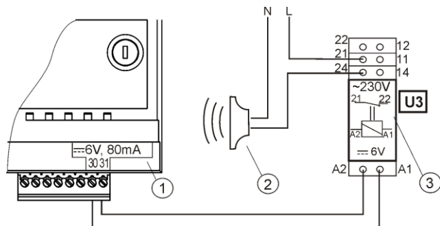
Rys. 40 Podłączenie zewnętrznego urządzenia alarmowego, gdzie: 1- regulator ecoMAX800, 2 - zewnętrzne urządzenie alarmowe, 3 - Moduł U3 składający się z przekaźnika RM 84-2012-35-1006 RELPOL i podstawki GZT80 RELPOL,
