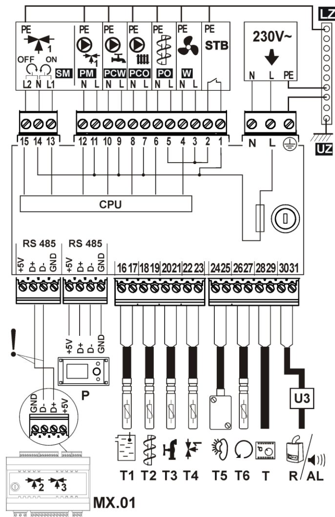
Rys. 31 Schemat połączeń elektrycznych z urządzeniami zewnętrznymi, gdzie: T1 - czujnik temperatury kotła CT4, T2 - czujnik temperatury podajnika paliwa CT4, T3 - czujnik temperatury ciepłej wody użytkowej, T4 - czujnik temperatury mieszacza pierwszego CT4, T5 - czujnik temperatury pogodowej typ CT4-P, T6 - czujnik temperatury wody powracającej do kotła (opcja), U3 - przekaźnik do podłączenia kotła rezerwowego lub alarmu, T - termostat pokojowy, R - kocioł rezerwowo, AL - sygnalizator alarmów, P - panel sterujący kotła, MX.01 -moduł rozszerzający (opcja, dwa dodatkowe obiegi grzewcze), ! - łączyć dwuprzewodowo - nie łączyć czterema przewodami. 230V~ - kabel zasilający, STB - ogranicznik temperatury bezpieczeństwa (rozłącza podajnik i nadmuchi), W - wentylator, PO- silnik podajnika paliwa, PCO - pompa centralnego ogrzewania, PCW - pompa ciepłej wody użytkowej, PM - pompa mieszacza, SM - siłownik mieszacza, LZ - listwa zerowa, UZ - uziemienie metalowej obudowy regulatora.
