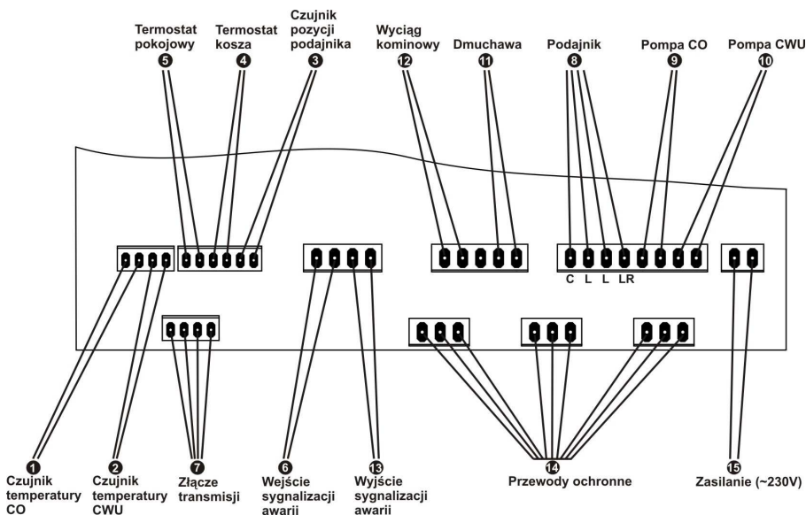
Rys. 2. Podłączenie współpracujących urządzeń.
