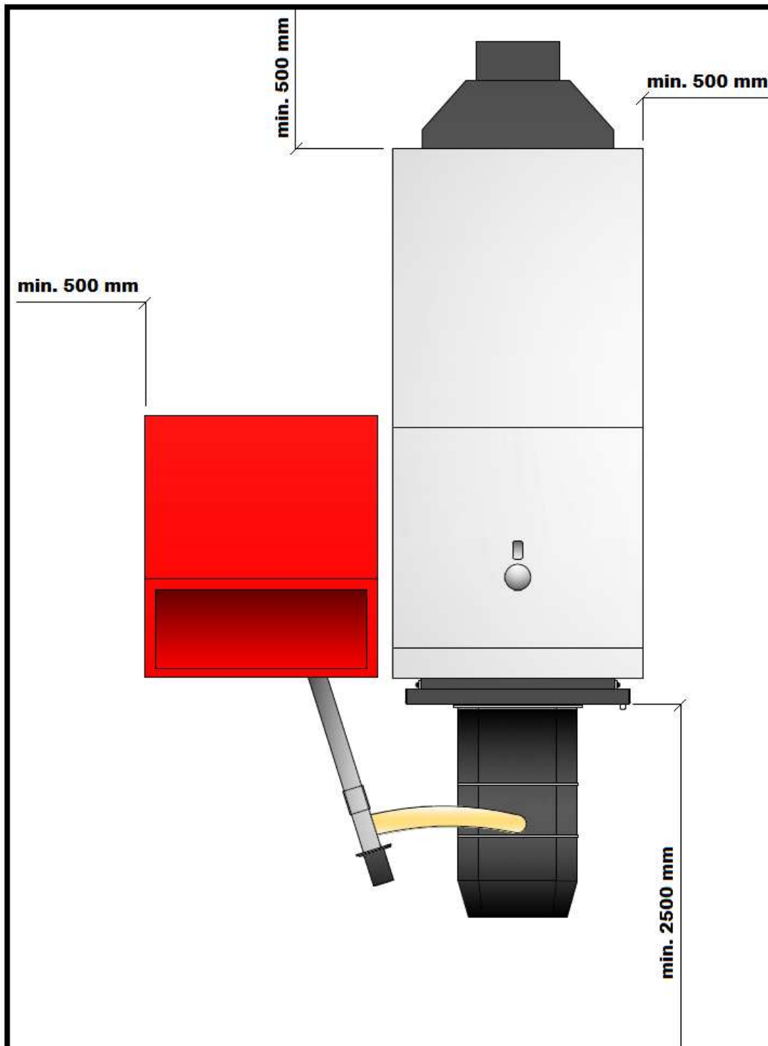
Przykładowy szkic sytuacyjny w kotłowni
