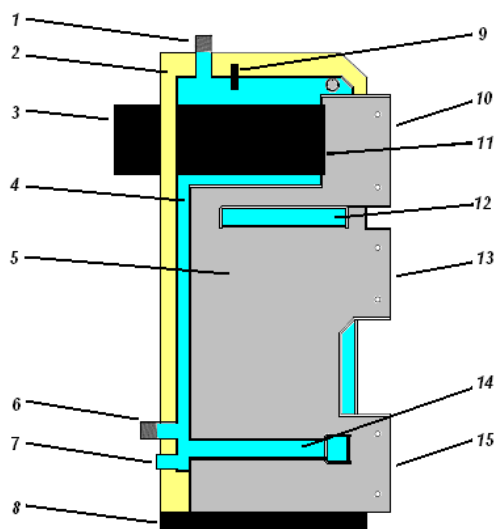
Rys. 1 Przekrój wzdłużny kotła KOLIBER 2.1 Podstawowe wymiary kotła
